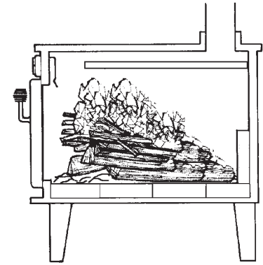
Figure 5 : Technique d'allumage inversée
