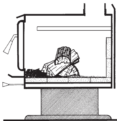
Figure 7 : Une petite charge de bûches entrecroisées pour temps clément
