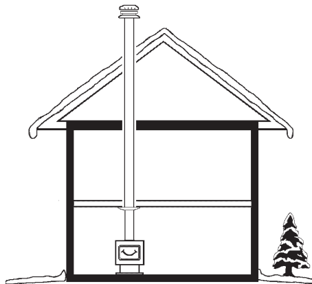
Figure 1 : La façon dont cette cheminée et son conduit de fumée sont disposés procure une performance optimale
