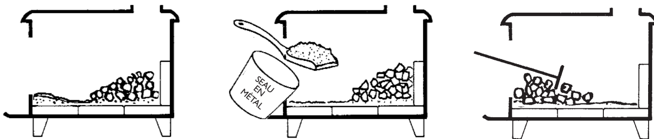
Figure 6 : À gauche, des charbons à l'arrière, de la cendre à l'avant; au centre, enlèvement de la cendre; à droite, charbons ramenés vers l'avant
