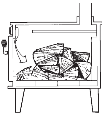
Figure 8 : Une charge orientée est-ouest
